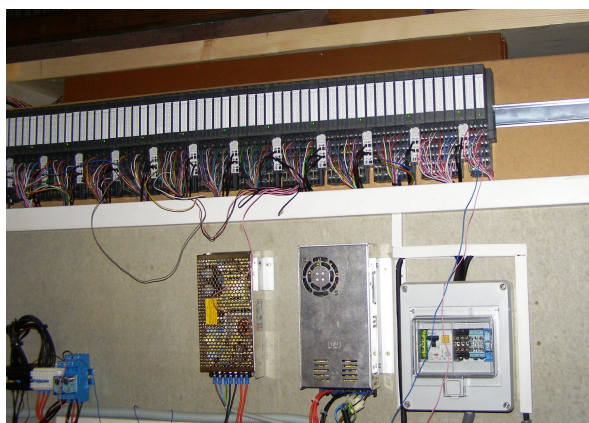
Panel s osazenými periferními ovládacími jednotkami a stabilizovanými zdroji
